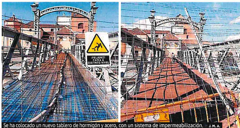
Se ha colocado un nuevo tablero de hormigón y acero, con un sistema de impermeabilización. J. M. A.
